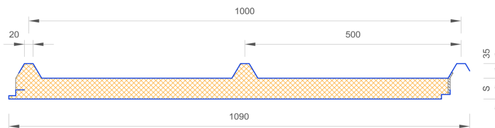
provedení : PUR fotovoltaický modul
